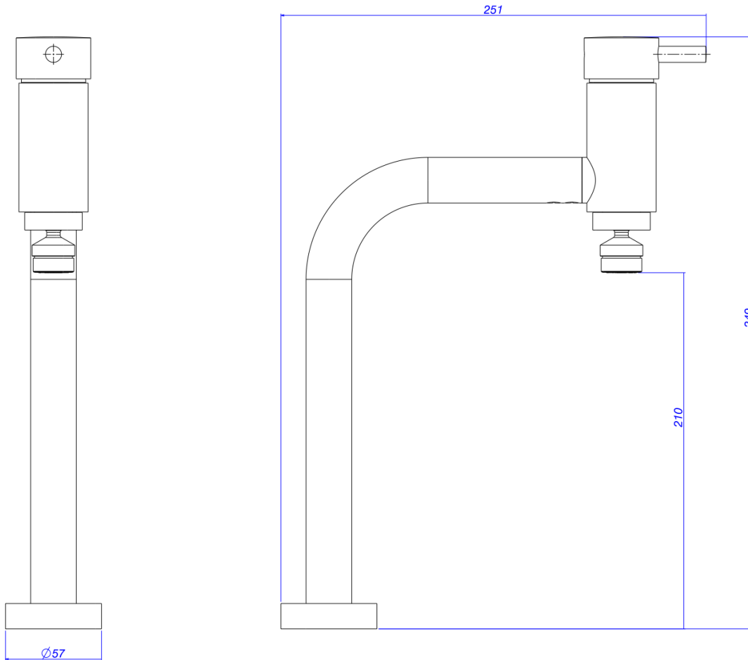
Desenho Técnico
